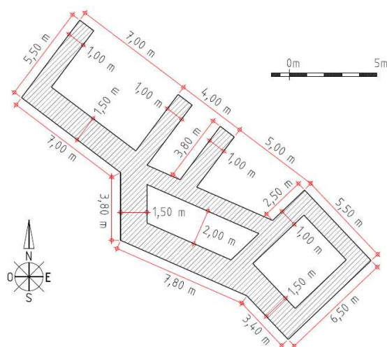
Plano de planta general de la construcción "C". (J. J. Ortuño-2020)
