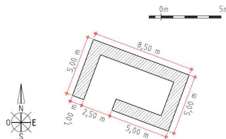
Plano de planta de la construcción “A”. (J. J. Ortuño-2020).
