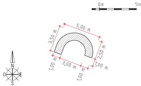
Plano de planta de la construcción “B”. (J. J. Ortuño-2020).
