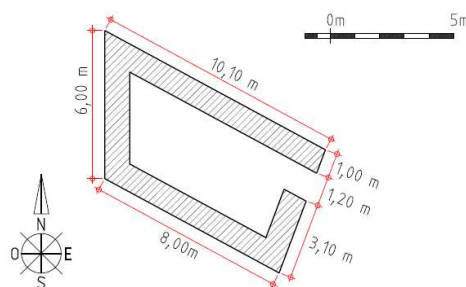
Plano de planta de la construcción "D". (J. J. Ortuño-2020).
