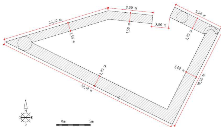
Pano de planta del recinto "E". (J. J. Ortuño-2020).
